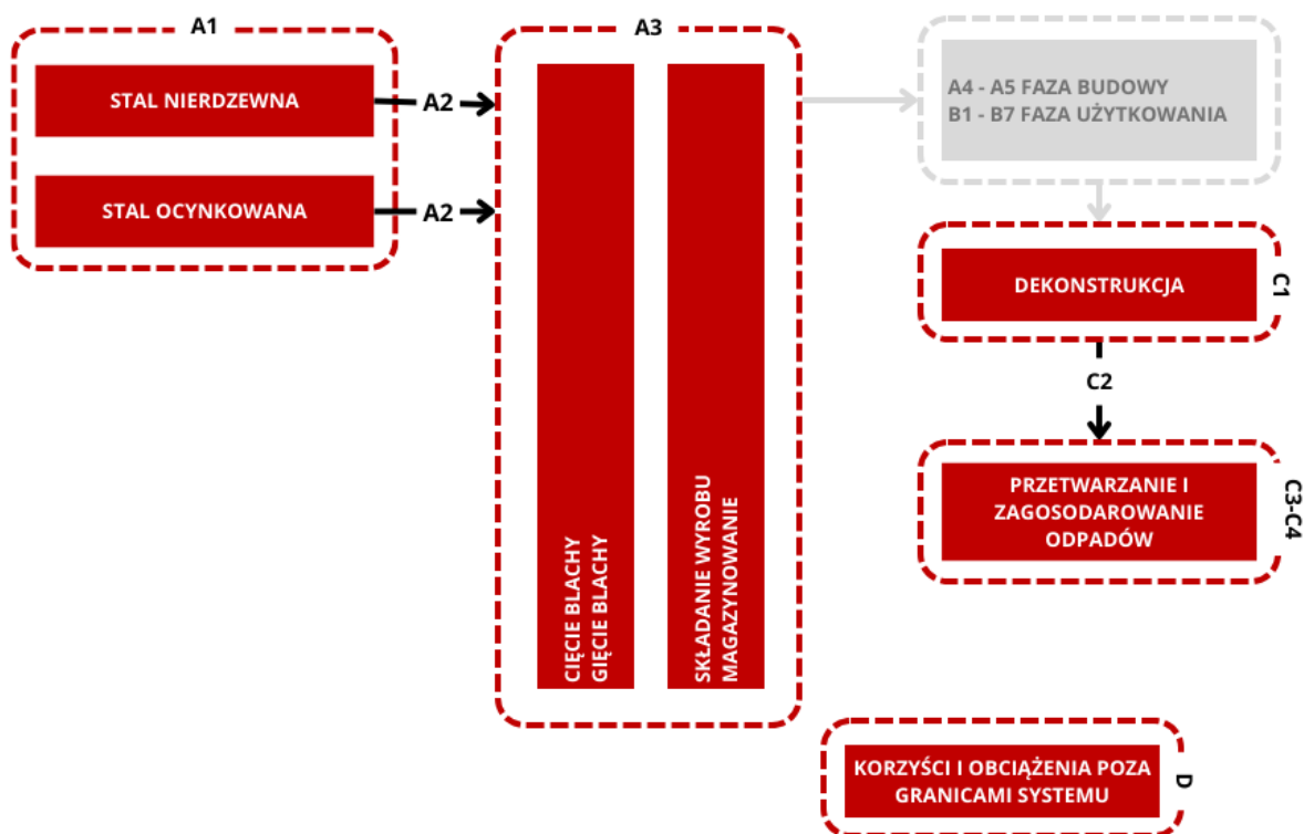
Rysunek 5.3: Granice systemu dla charakterystyki środowiskowej kratki stalowej do grzejników
