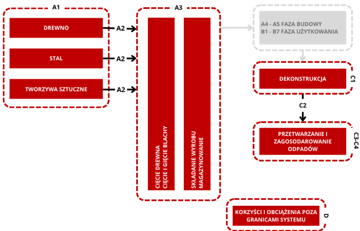
Rysunek 5.2: Granice systemu dla charakterystyki środowiskowej kratki drewnianych do grzejników
