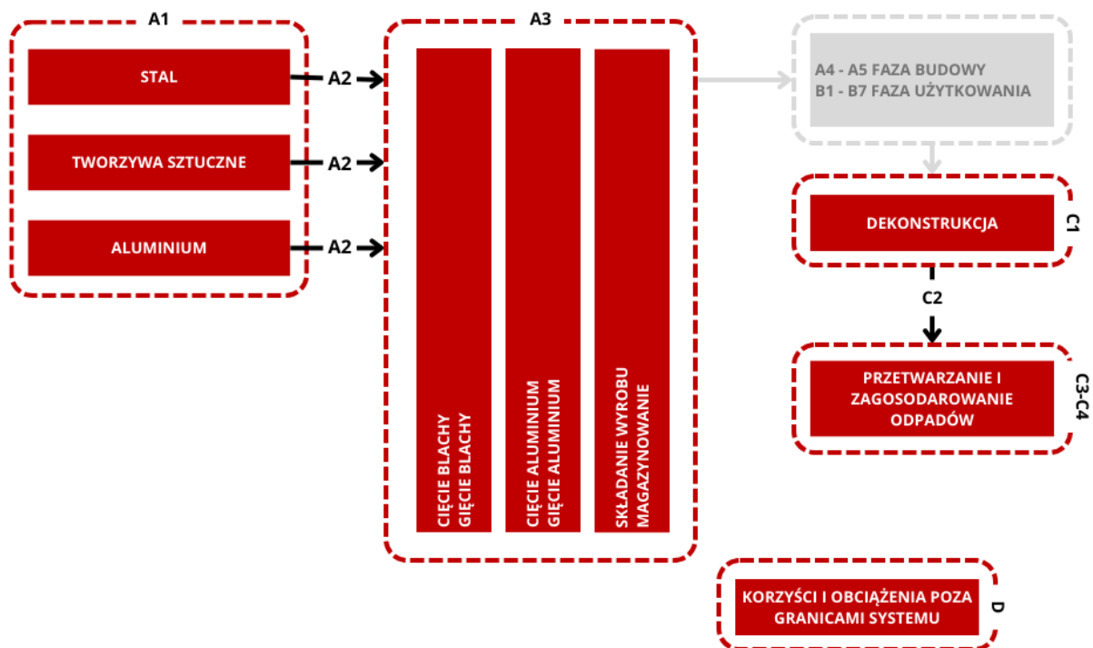
Rysunek 5.1: Granice systemu dla charakterystyki środowiskowej kratki aluminiowych do grzejników
